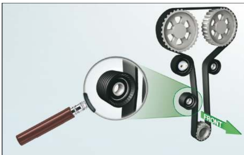
Рис. 1: Траектория ремня и позиция ролика на двигателе F4R
