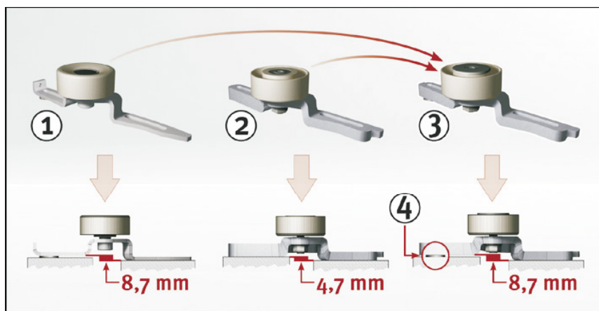
Рис. 1: Иллюстрация натяжных роликов и их разница.
