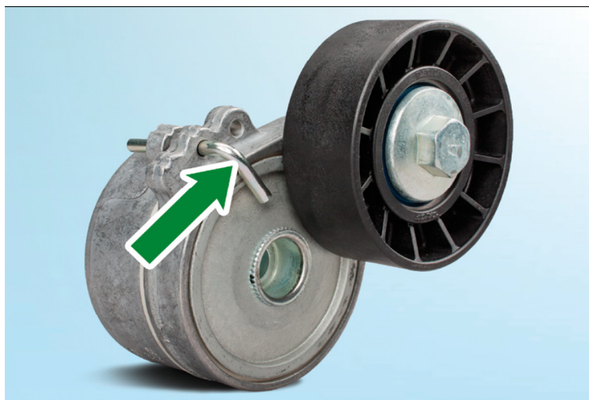
Рис. 1: 534 0110 20 — Натяжитель INA с фиксирующим штифтом
