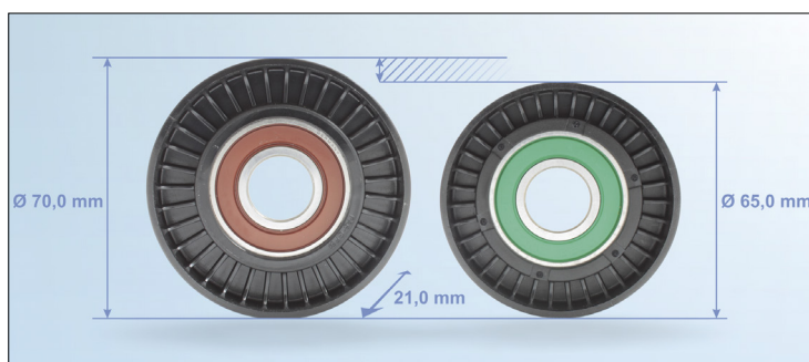
Рисунок 2: Направляющий ролик 532 0404 30 (слева) и направляющий ролик 532 0406 30 для дизельных двигателей (справа)
