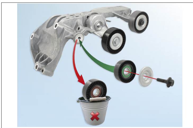
Рисунок 1: Натяжной узел 534 0243 10
