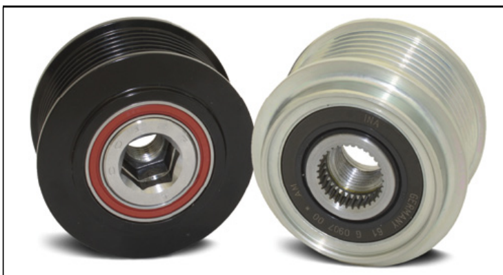
Рис. 2: При установке шкива генератора с обгонной муфтой на генератор Visteon (Ford Mondeo III) необходимо использовать прокладку толщиной 3 мм!
