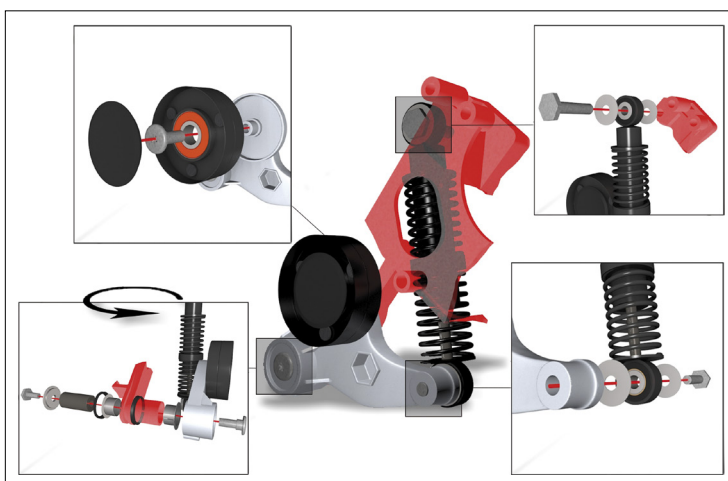
Рисунок 2: Обзор крепежных частей
