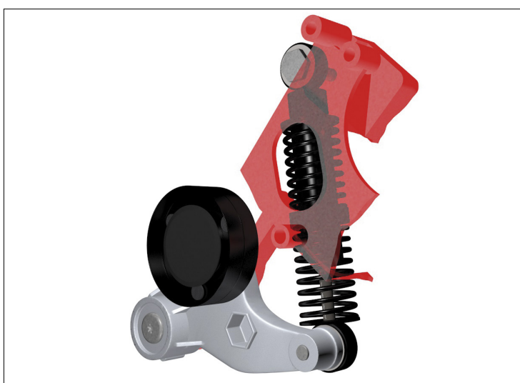
Рисунок 1: Натяжной модуль в сборе
