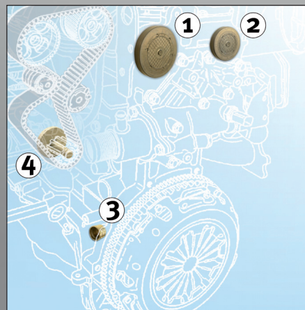
Рис. 2: Пункты монтажа
