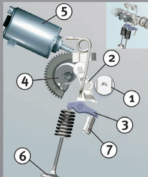
Илл. 1: общий вид BMW-Valvetronic / детальный вид компонентов системы
