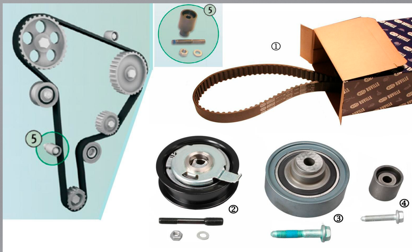
Рис. 1: схема привода 1.9 TDI/SDI и содержимое упаковки ремкомплекта 5549173/5549170, увеличенный вид см. стр. 2
