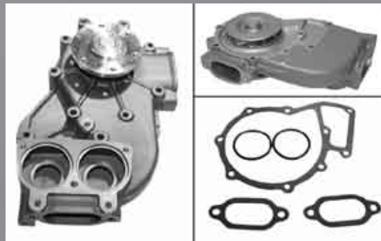
Илл. 1: Водяной насос 65136 (без термостатов)
