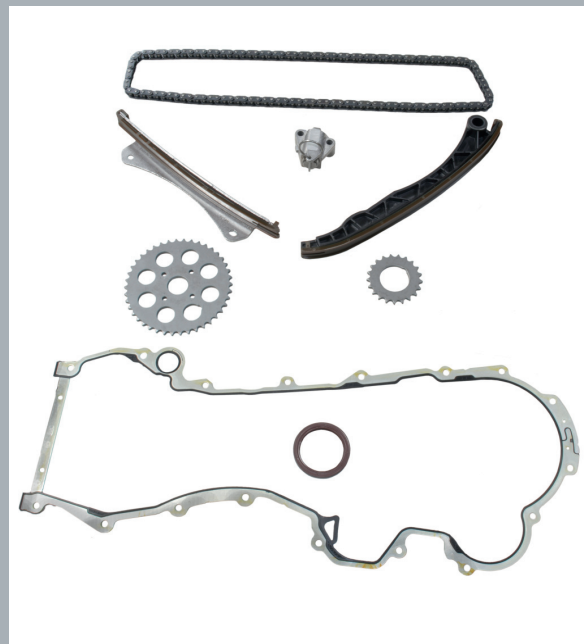
Илл. 1: 3458010SD, полный комплект с уплотнениями
