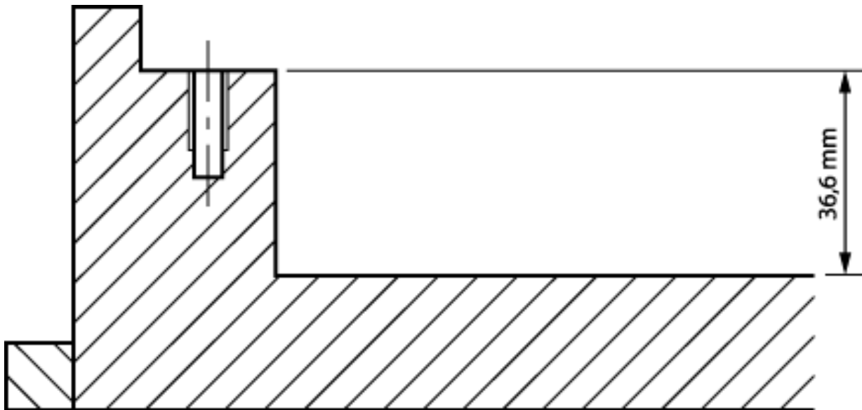
Abb./ Fig. 1: Schwungrad / Flywheel / Volant Moteur / Volante del motor
